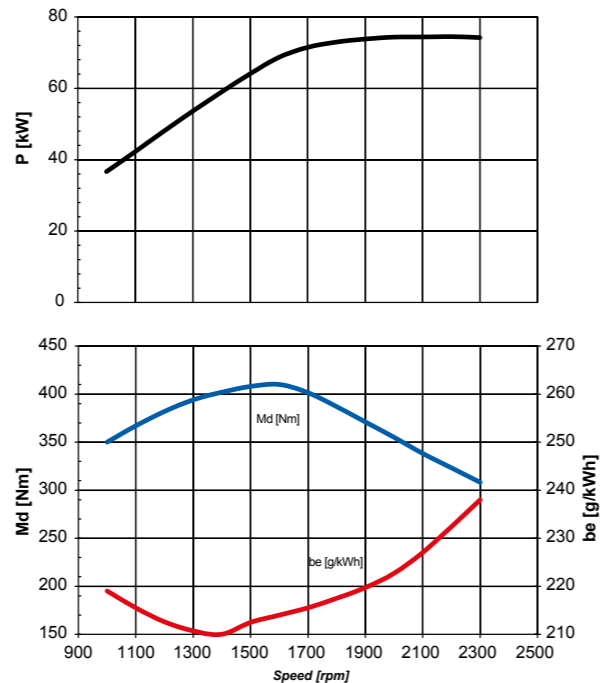
7.63C Deutz TCD 3.6 L4 78 kW - 106 CV
